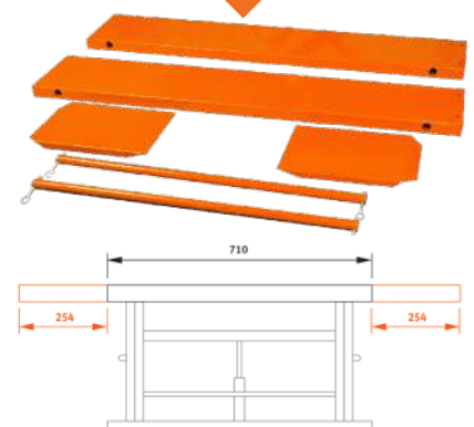
MHB 680 com extensão lateral
