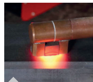
Aquecimento de um componente com a bobina de foco em linha recta
