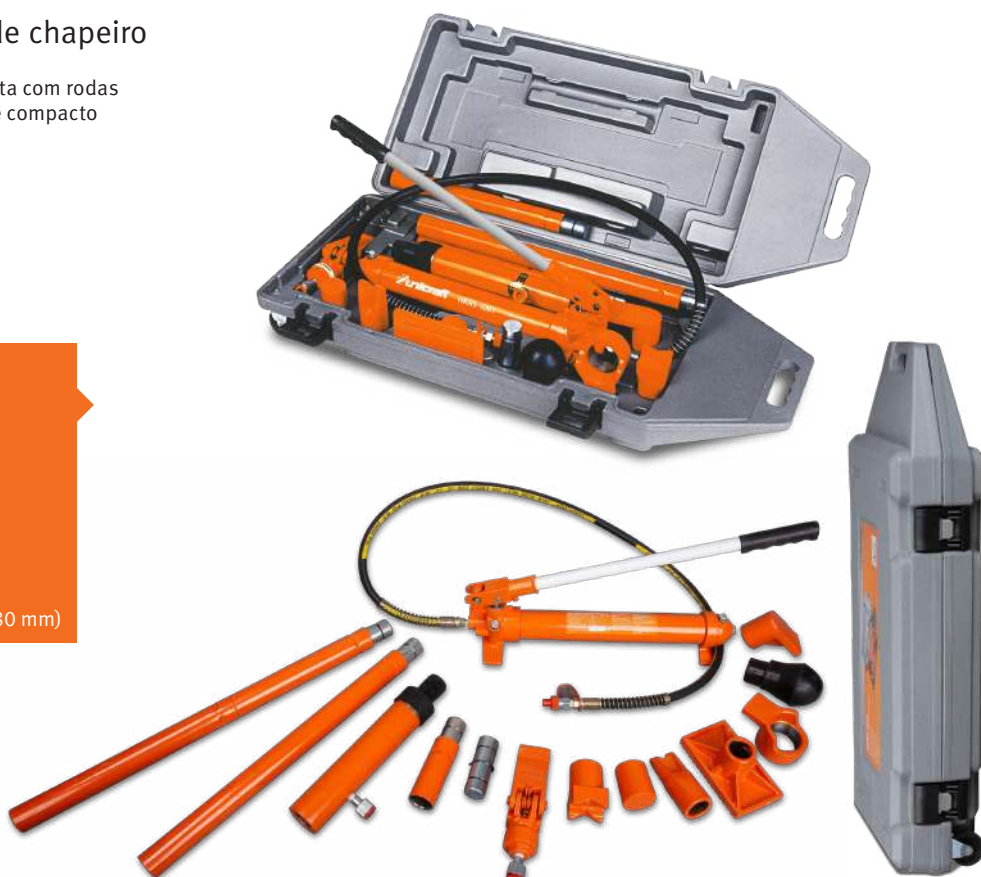
Caixa de plástico resistente com rodas
