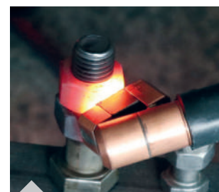
Aquecimento de uma porca com bobina de foco em ângulo
