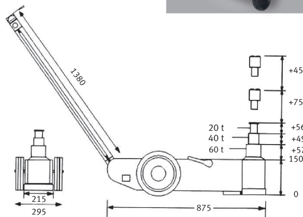
WWH 60000 PH Dimensões e capacidade de carga
